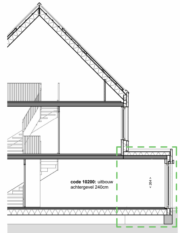
doorsnede
