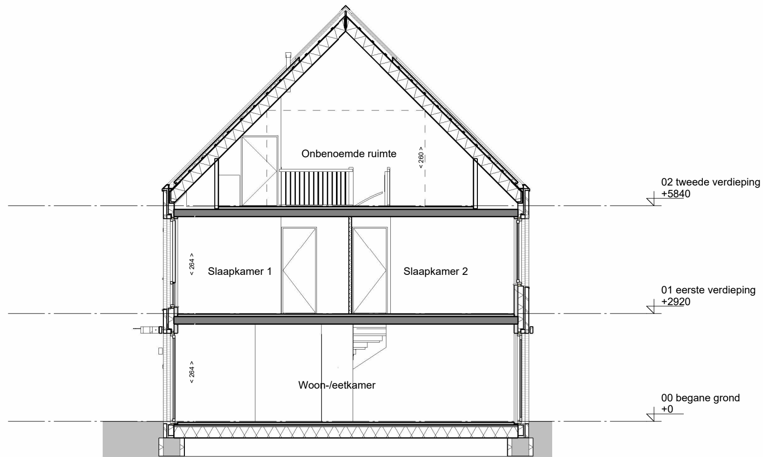
doorsnede
