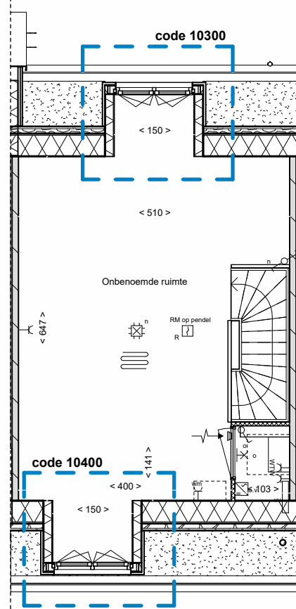
achtergevel
