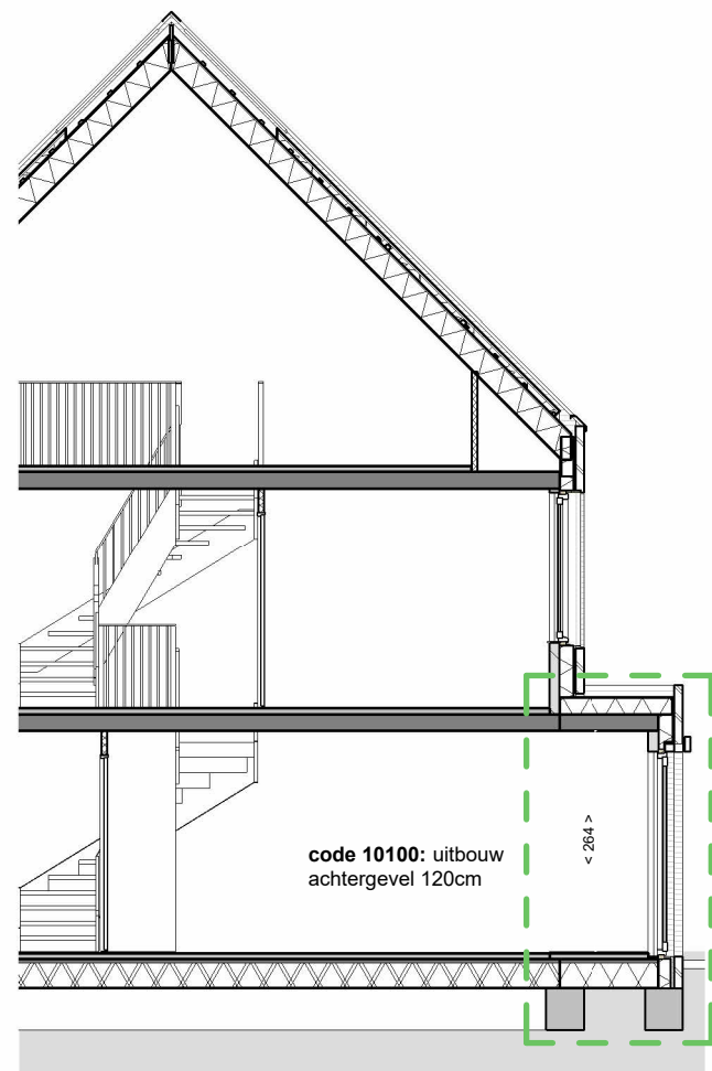
doorsnede
